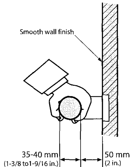
Figure 4.2.10.1 Grab Bar
