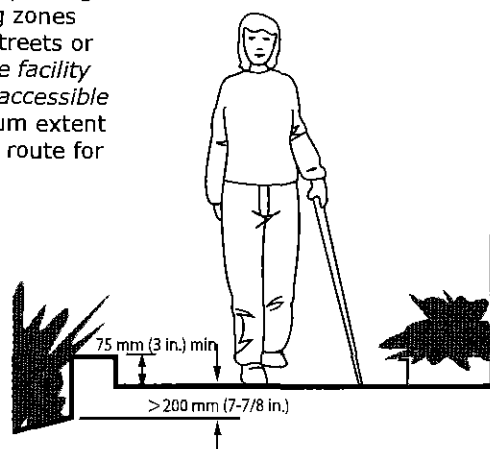
Figure 4.1.4.1 Edge Protection
